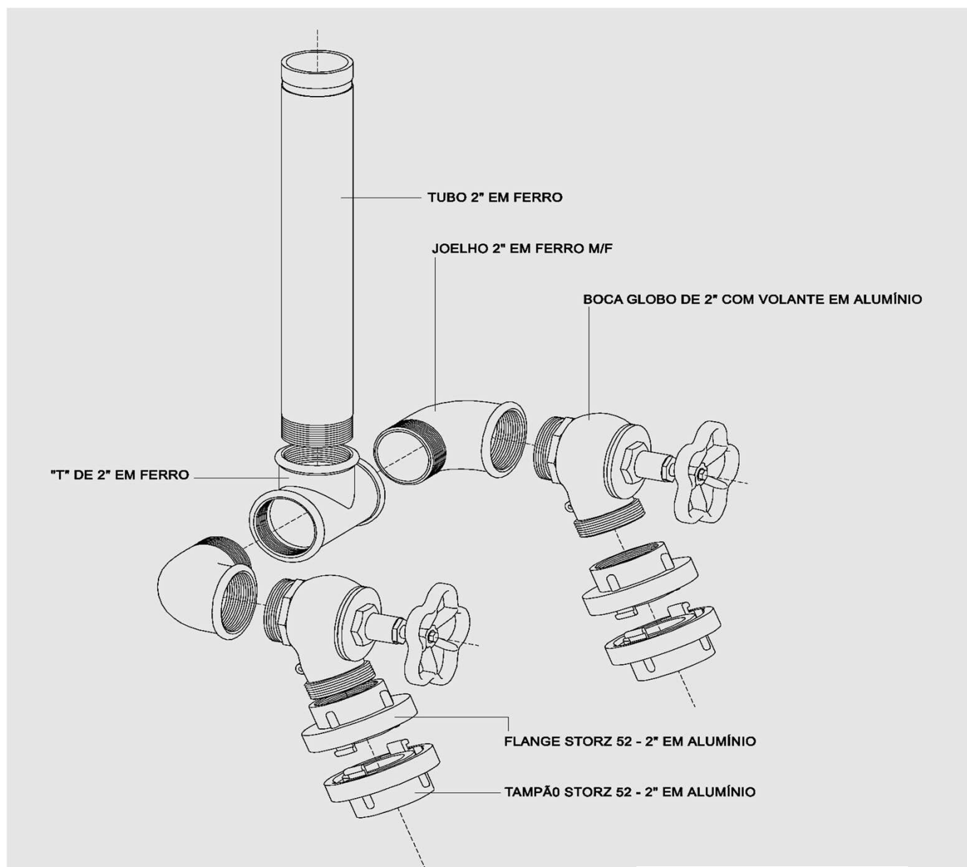
AXONOMETRIA EXPLODIDA
